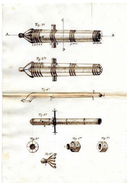
Dibujo del proyecto para fabricar cañones de hierro forjado (1809), del Archivo General Militar de Segovia.
