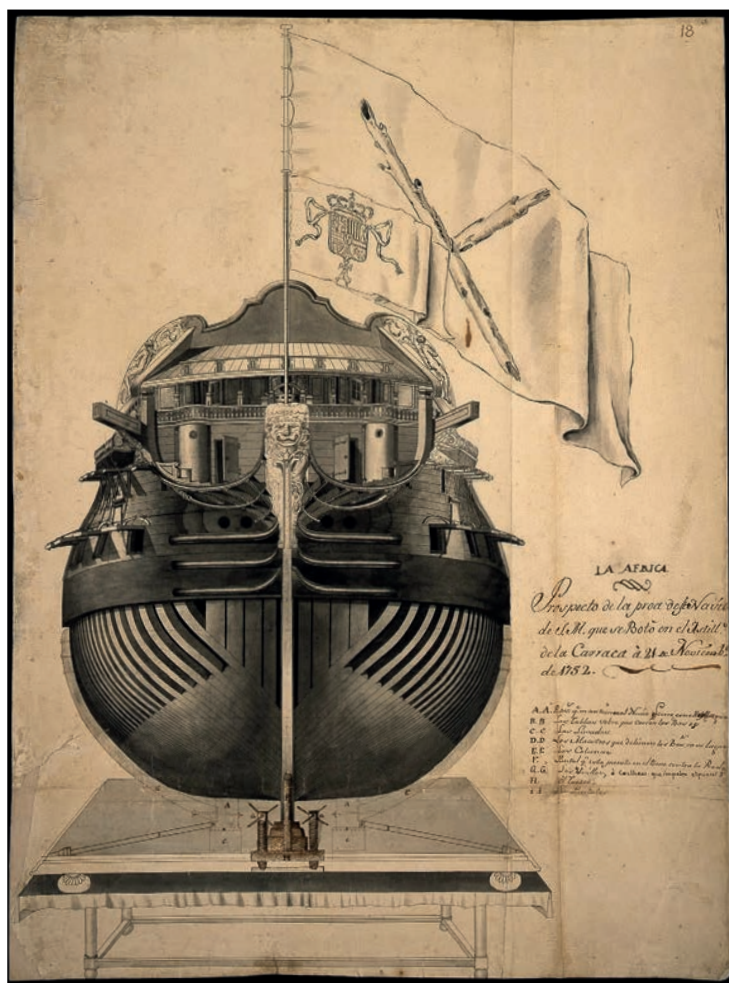
Prospecto de la proa del navío La África , A. Museo Naval (Madrid).
